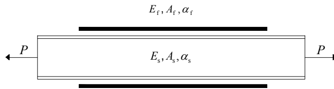
Figura 6-5 – Calcolo di \Delta\varepsilon_{fs} nel caso di un elemento metallico teso, rinforzato in modo simmetrico e soggetto ad una forza assiale P e ad una variazione di temperatura uniforme \Delta T .
